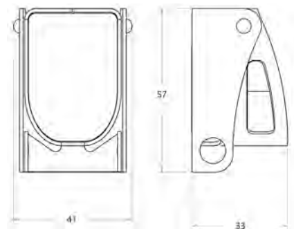
Schlossabdeckung
