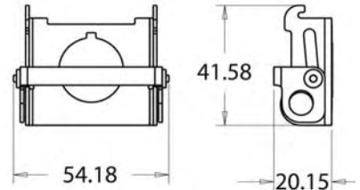
Abschließvorrichtung für tastende Pilztaster
