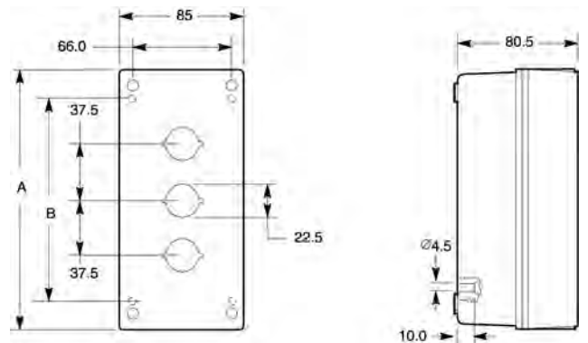
Metallgehäuse
