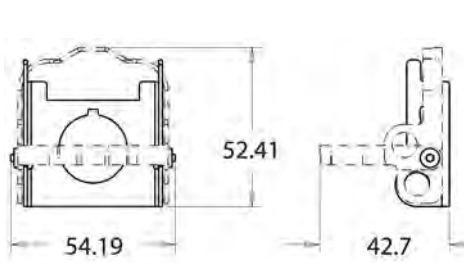
Abschließvorrichtung für rastende Pilztaster
