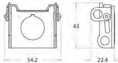
Erhöhte Abschließvorrichtung, unbeleuchtet
